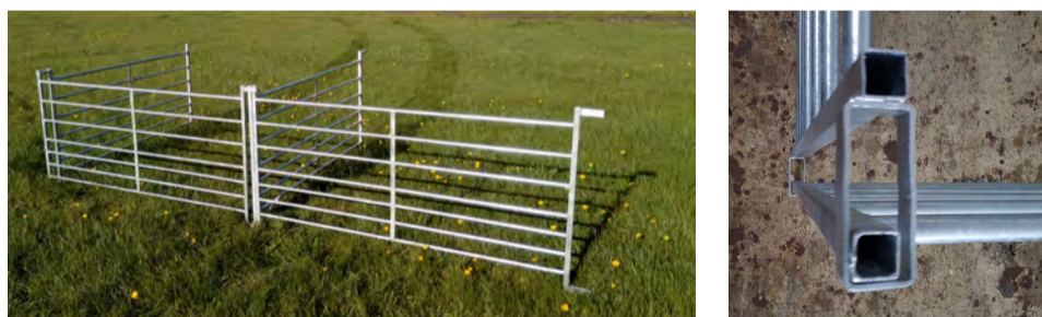
Liprar og léttar fjárgrindur. Krækt saman án aukahluta. Breidd 180 cm, hæð 90 cm.
